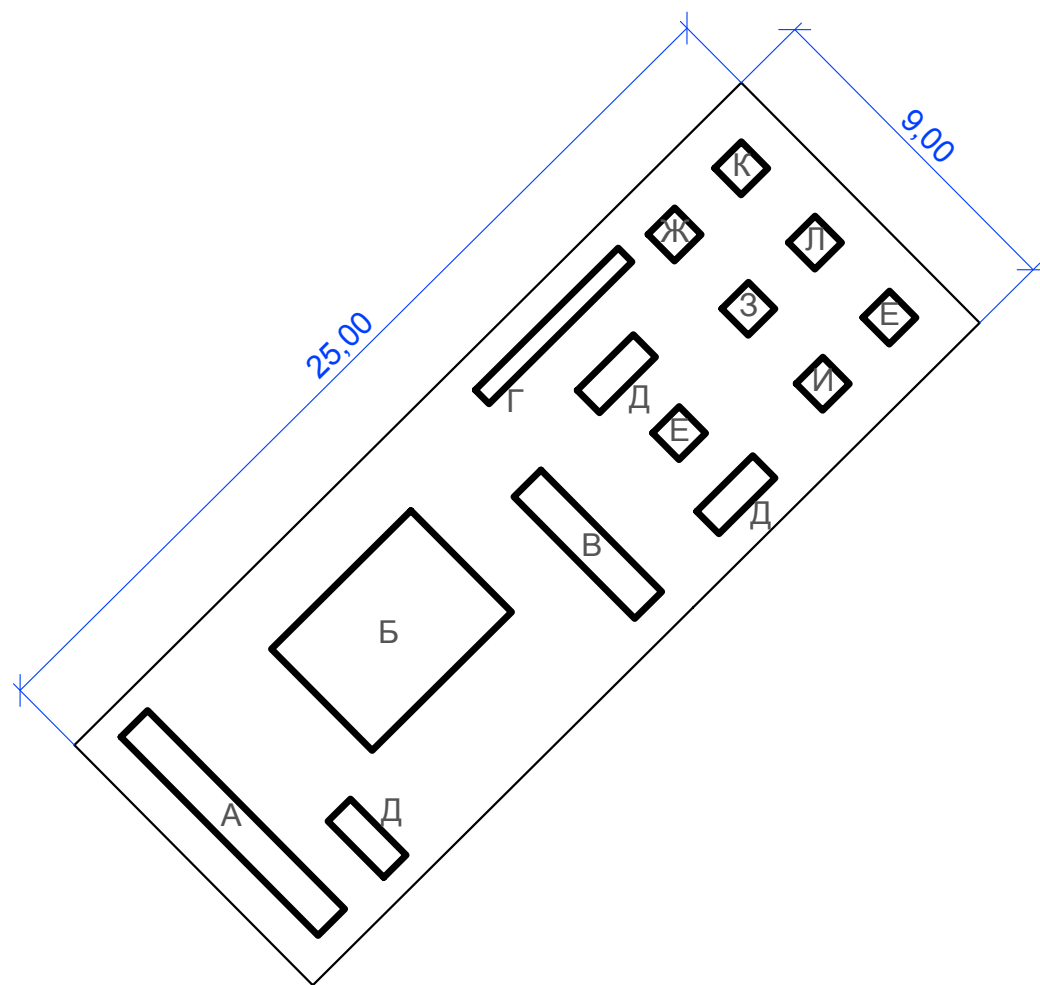
Спортивная площадка 1. М1:200
